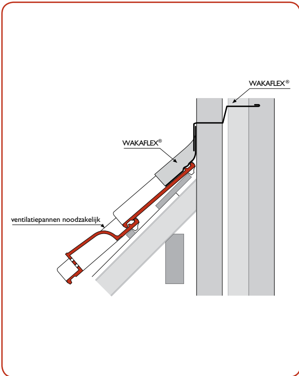
Muuraansluiting (verticaal)
