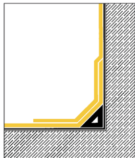
Cant Strip op niet-geïsoleerde dakvloer
