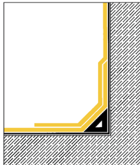
Cant Strip sur support non isolé
