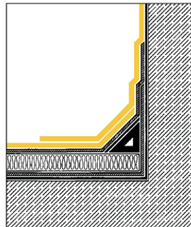
Cant Strip sur isolant avec étanchéité bicouche
