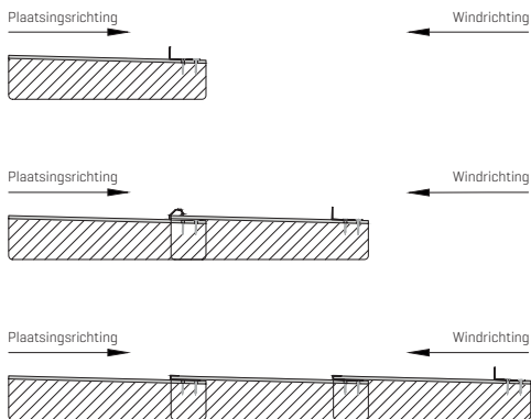
Plaatsingsrichting nokken
