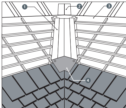
Gesloten ki(e)lgoot
