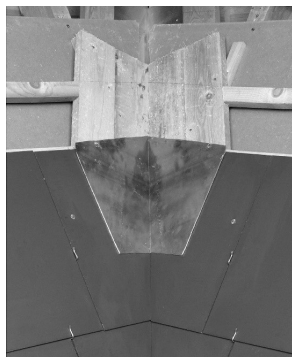
Gesloten ki(e)lgoot
