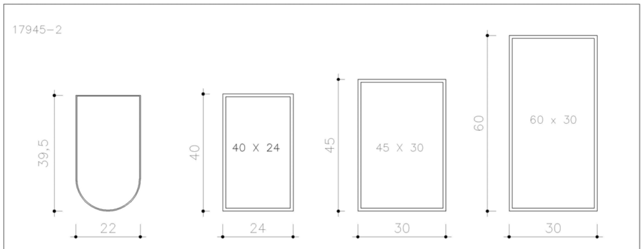
Fig. 3: Dimensions des ardoises NEW STONIT et/ou UMBRA en cm
