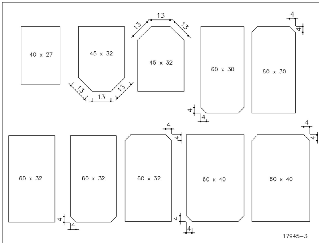
Fig. 2: Dimensions des ardoises ALTERNA et/ou BORONDA et/ou ACTIVA en cm
