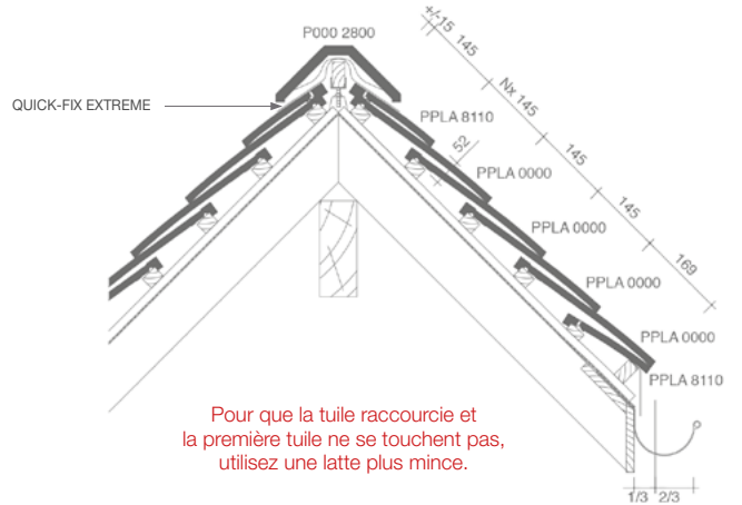
PLAN DE POSE LONGITUDINALE DE LA TOITURE AU NIVEAU DE LA FAÎTIÈRE 2800 - AVEC QUICK-FIX EXTREME
