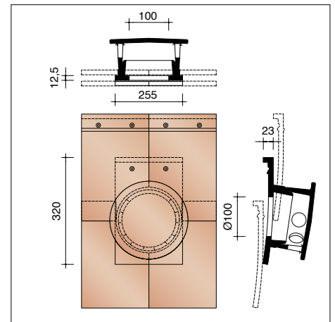
PPLA8961 Kit tuile à douille Ø 100 mm + mitron - 95 cm 2 + module de connexion
