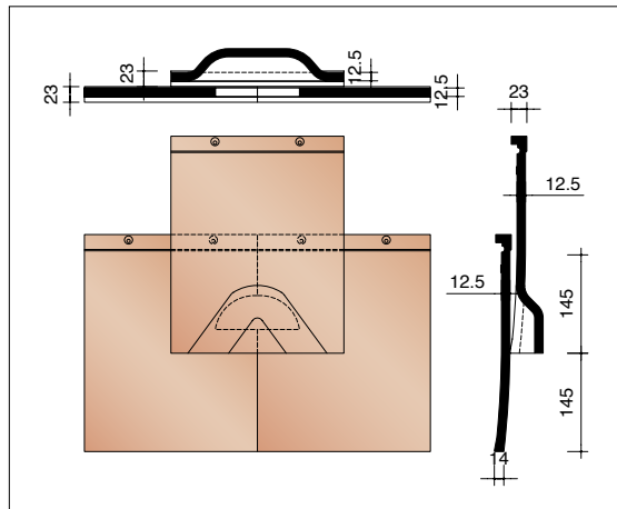
PPLA8611 Kit de ventilation avec grille - 43 cm 2
