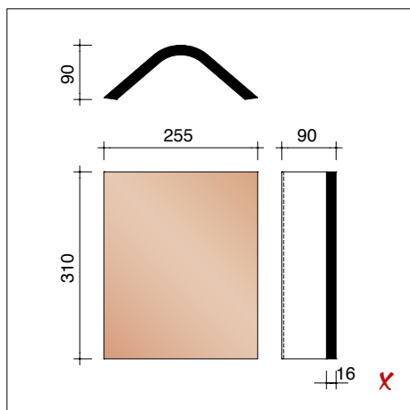
K0001800 3,3 pièces/m crt Faîtière angulaire
