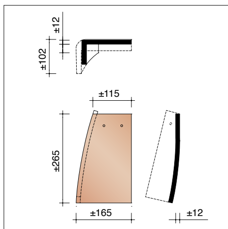
KSHI/KGOX 8800 4,2 pièces/m crt Pièce d'angle gauche (bardage)
