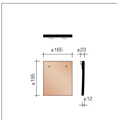
KSHI/KGOX 8110 6 pièces/m crt Tuile raccourcie
