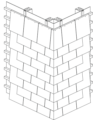
* DESSIN 3D BARDAGE AVEC COUPE
