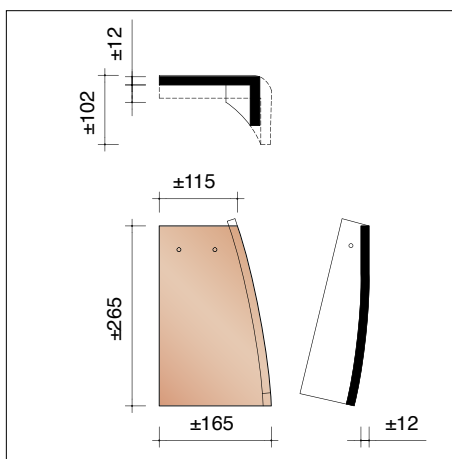
KSHI/KGOX 8810 4,2 pièces/m crt Pièce d'angle droite (bardage)
